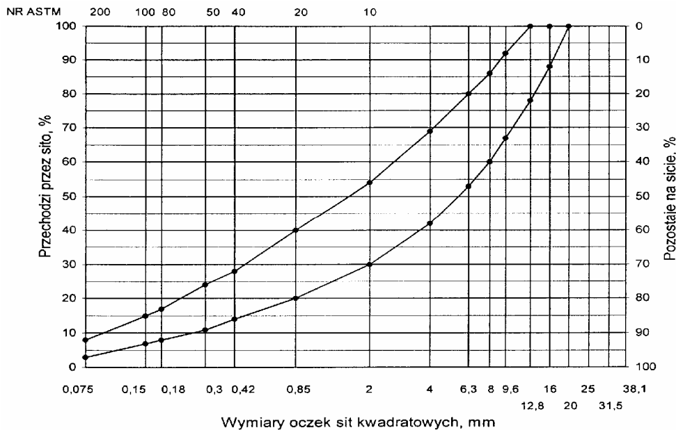
Rys. 8. Krzywe graniczne uziarnienia mieszanki mineralnej BA od 0 do 16 mm do warstwy wiążącej nawierzchni drogi o obciążeniu ruchem KR2
