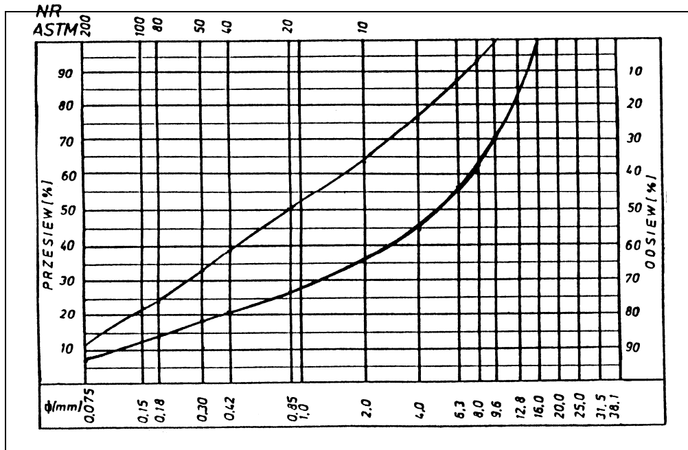
Rys. 2. Krzywe graniczne uziarnienia mieszanki mineralnej 0÷12,8 mm do warstwy wiążącej, wyrównawczej i wzmacniającej z betonu asfaltowego dla KR 1-2
