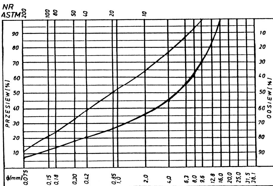
Rys. 1. Krzywe graniczne uziarnienia mieszanki mineralnej 0÷16, 0÷11,2 mm do warstwy ścieralnej z betonu asfaltowego dla KR 1-2
