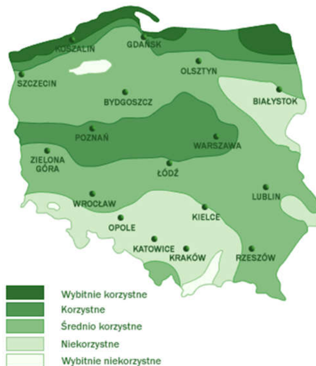
Rysunek nr 40. Mapa zasobów wietrznych IMGW
