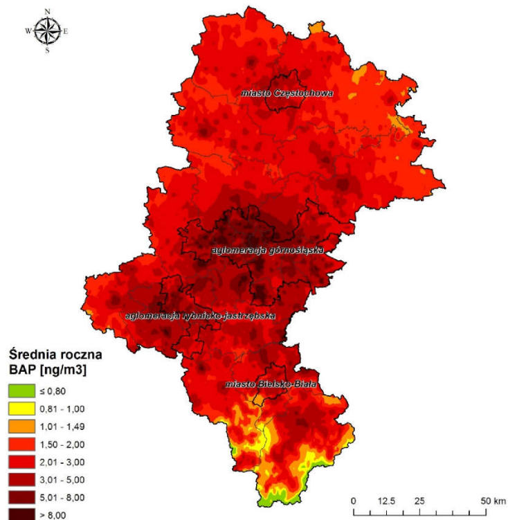
Rysunek nr 13. Obszary przekroczeń średnich stężeń rocznych benzo(a)pirenu
