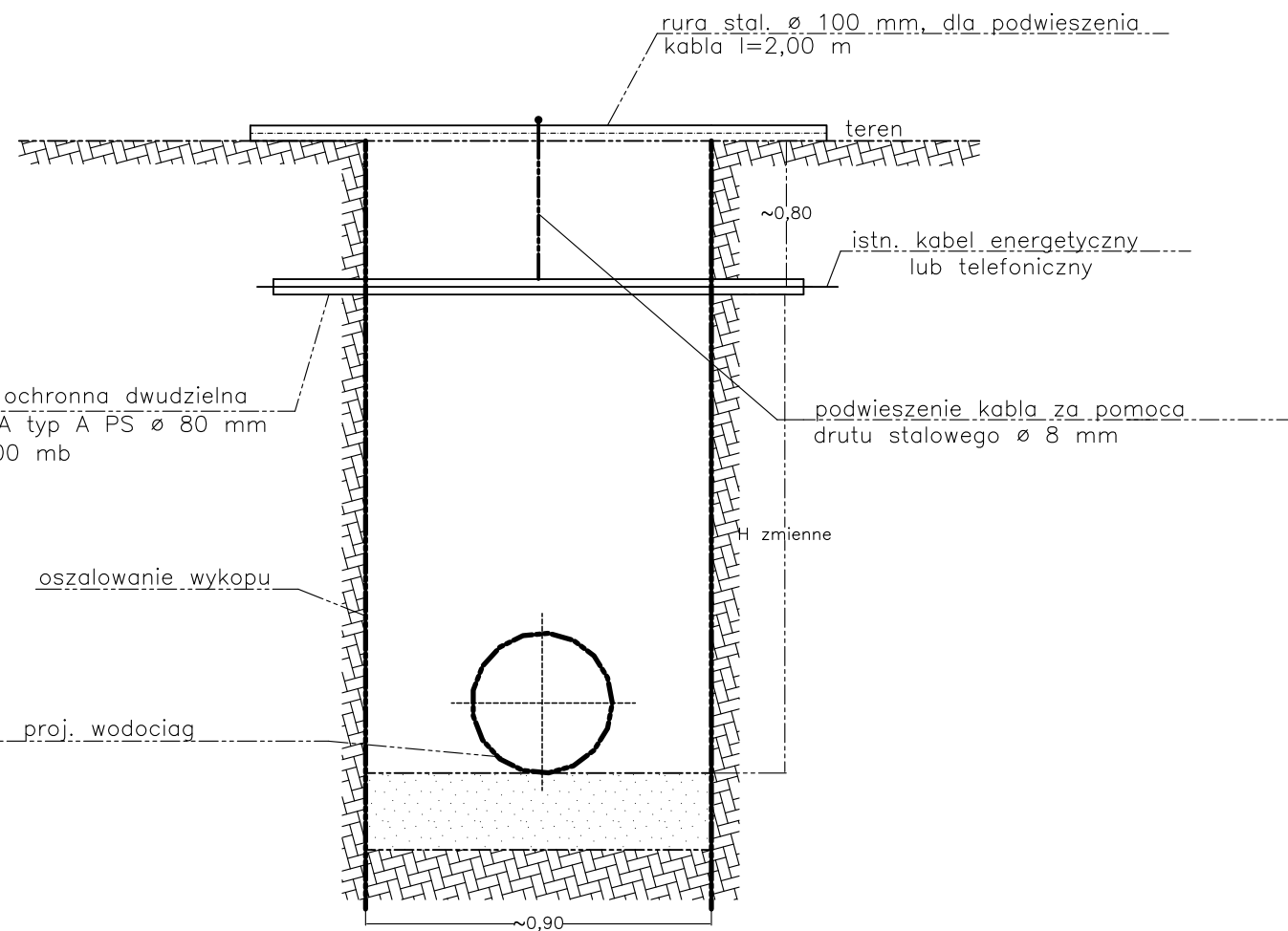
PRZEKROJ A-A
